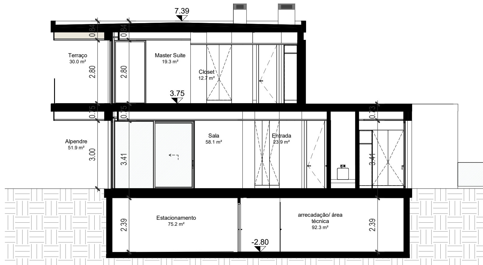
Corte Longitudinal
