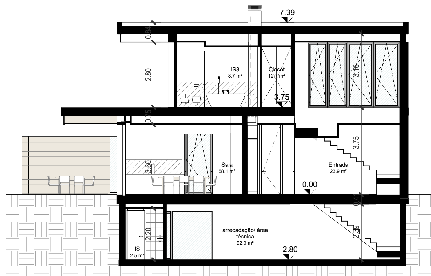
Corte Transversal
