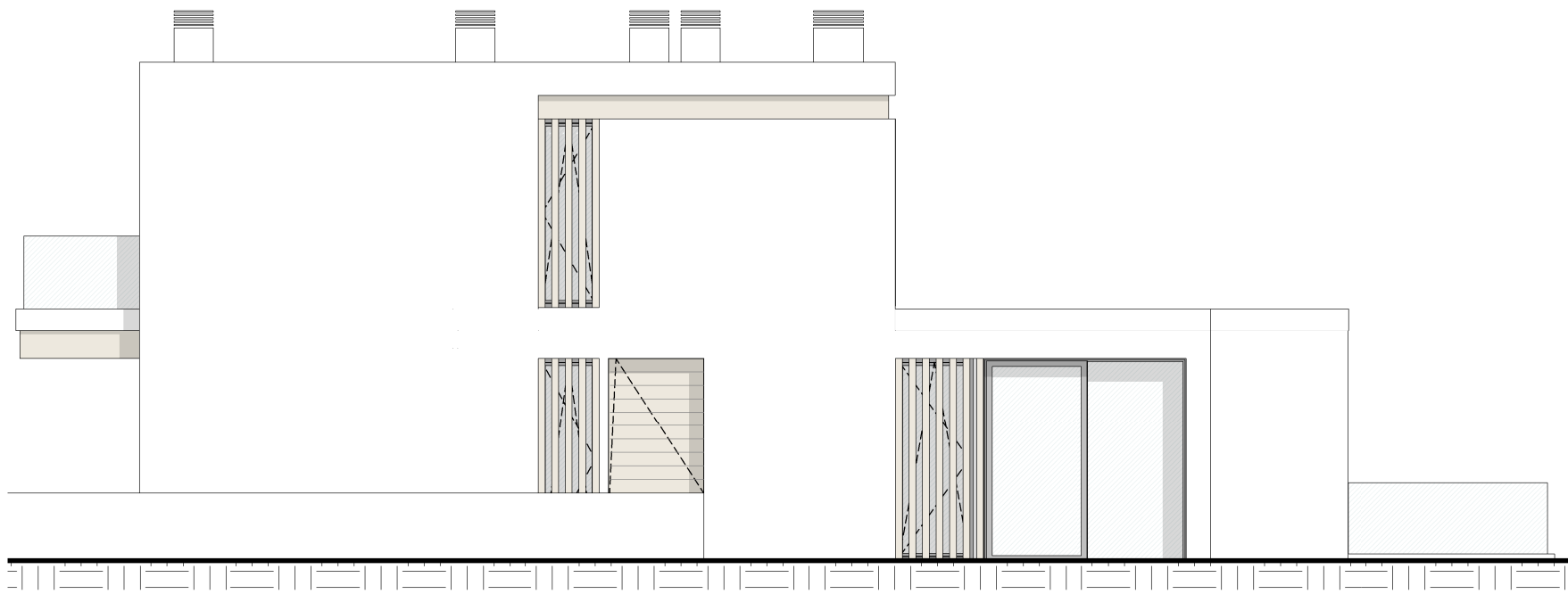
Alçado Nascente
