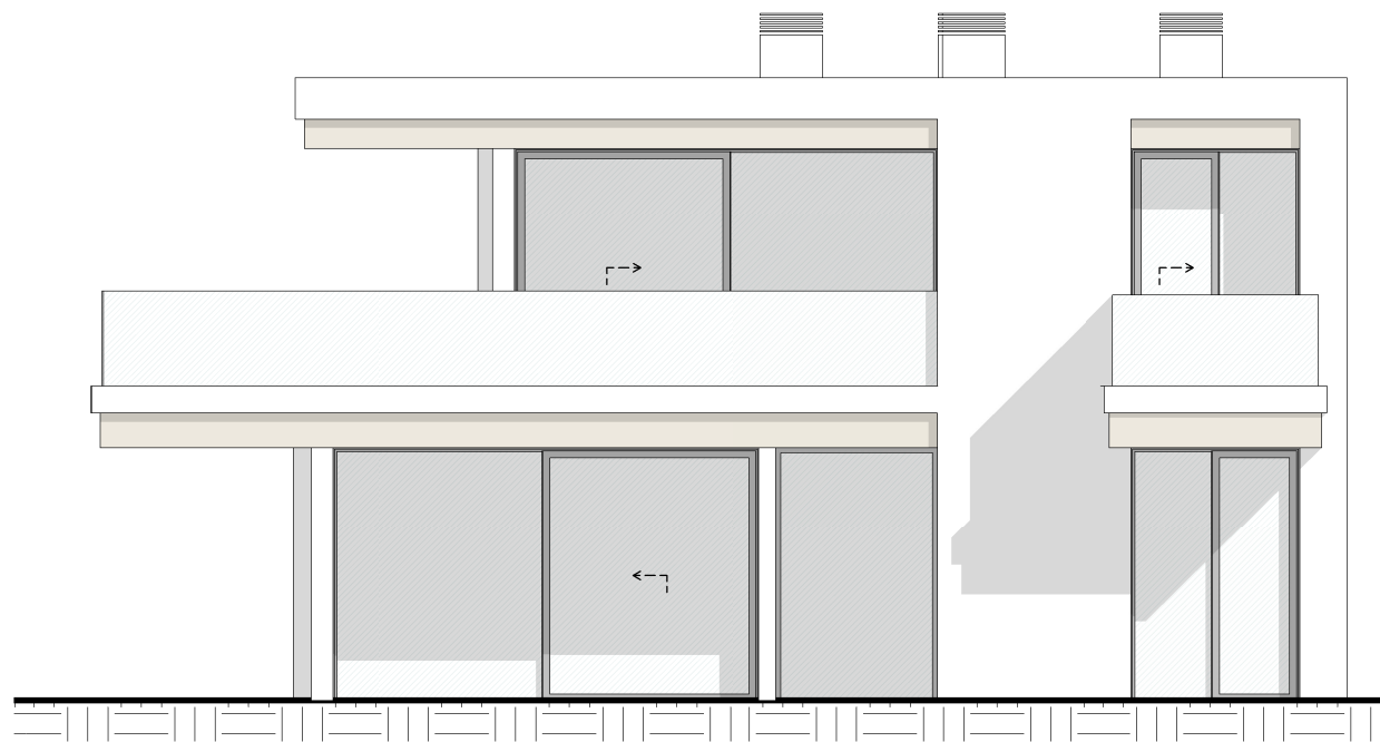
Alçado Sul
