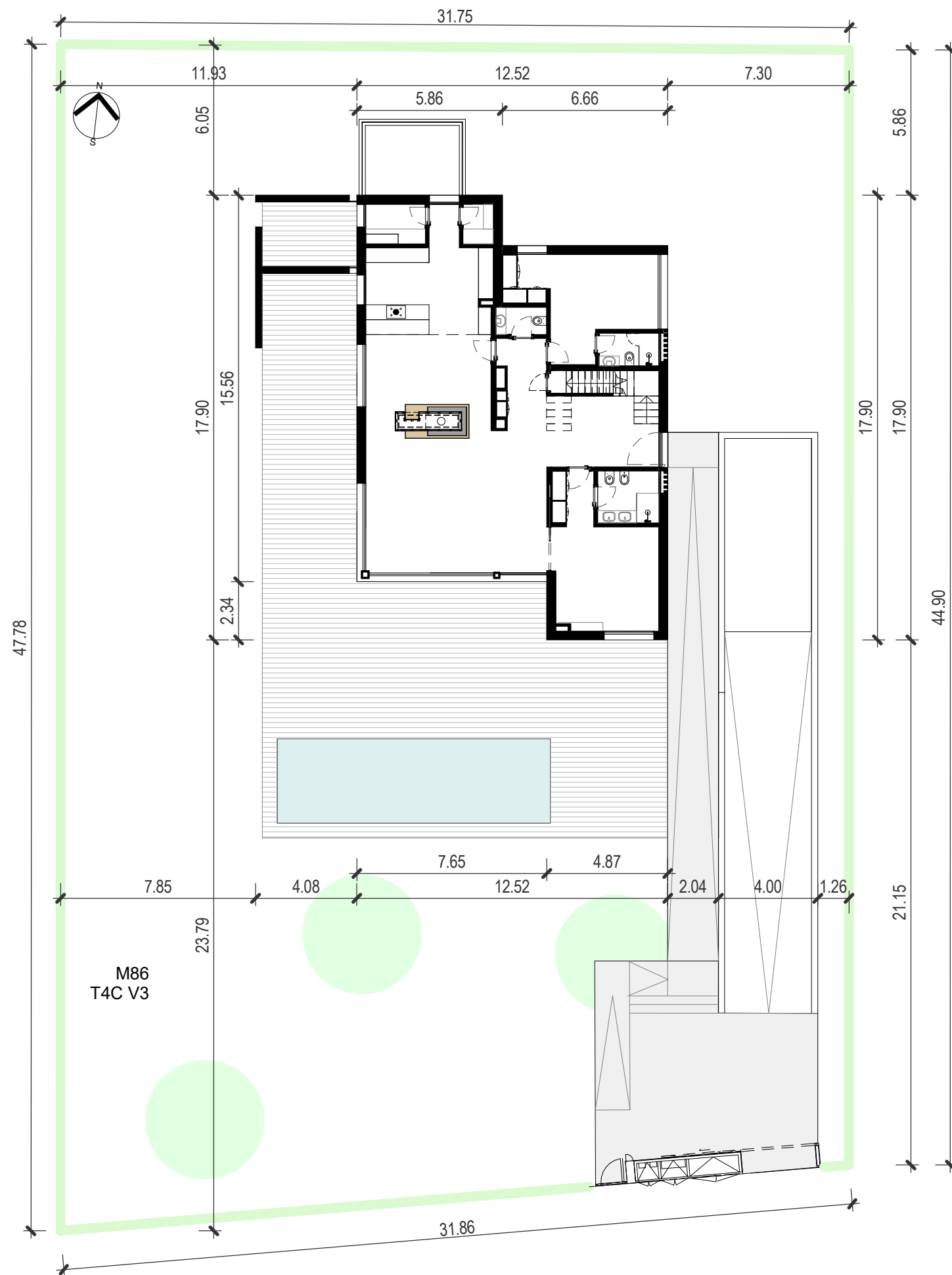
PLANTA DE IMPLANTAÇÃO M86
